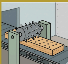
2. インサイジング
